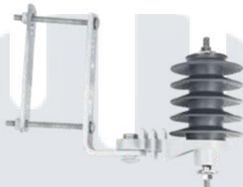
SECCIONADOR SWITCH TIPO ALTD CON AISLADOR ESP
